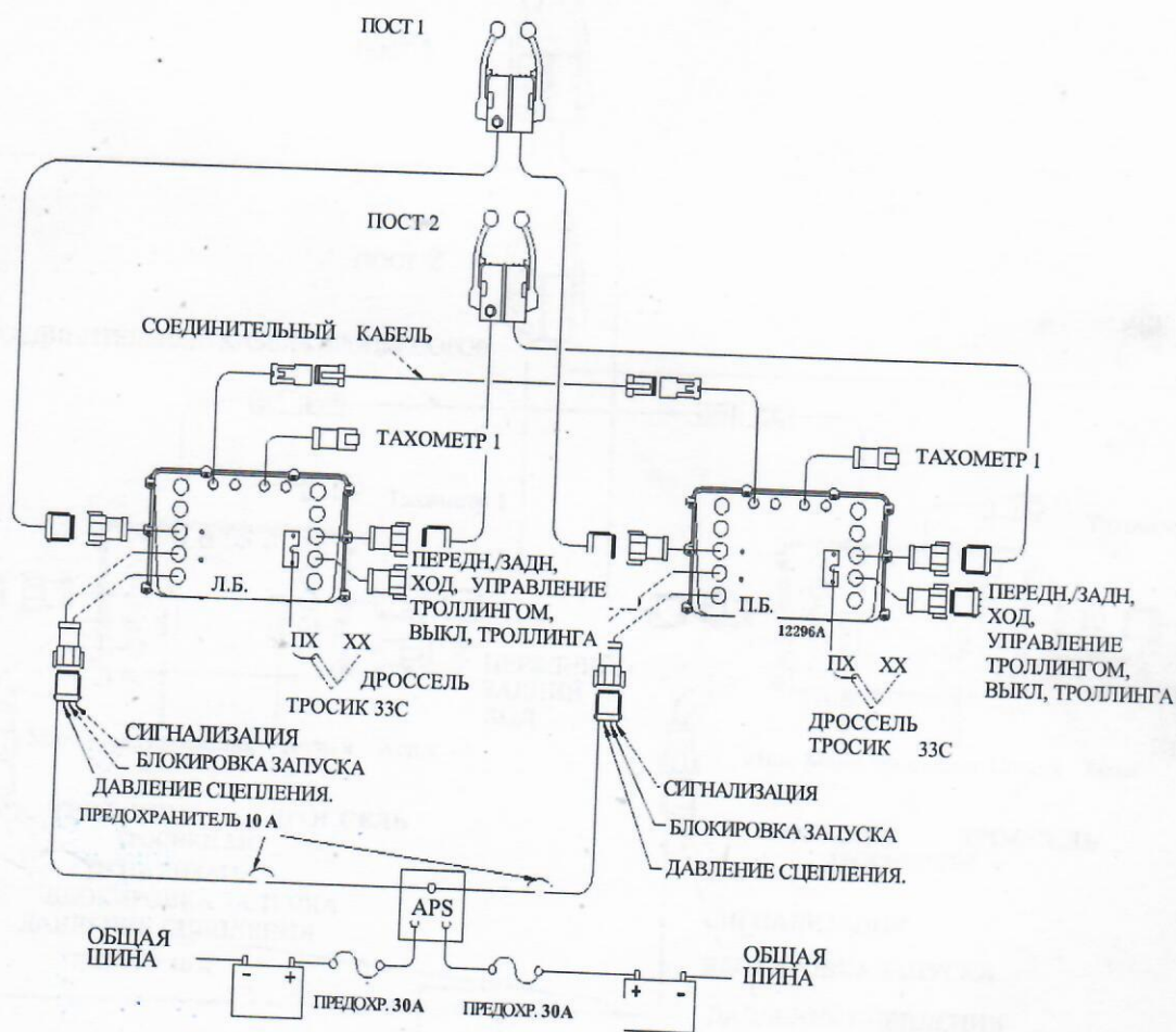
Рисунок 1-1: Схема системы ClearCommand 9120 или 9122, базовая версия
